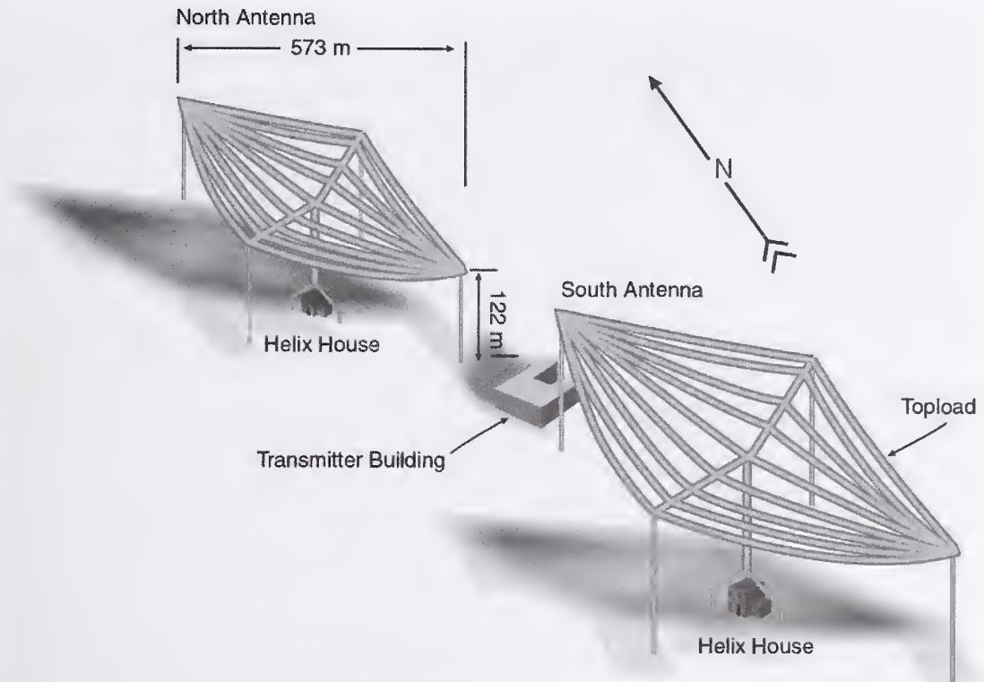
Figure 1.19. WWVB antennas.
